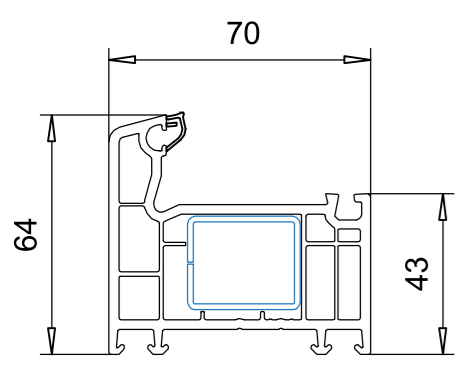
101.286 підсилювач 113.010 / 113.302
