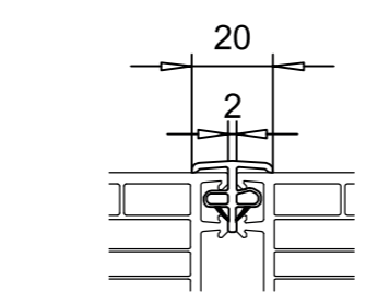
116.217 Міні з ʼєднувач
