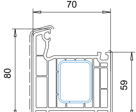
101.214 підсилювач 113.271 / 113.302
