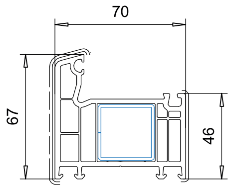
101.208 підсилювач 113.025
