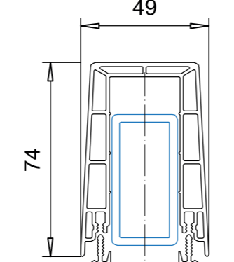
накладка 114.051 основа 114.050 підсилювач 113.161.3/113.398.3
