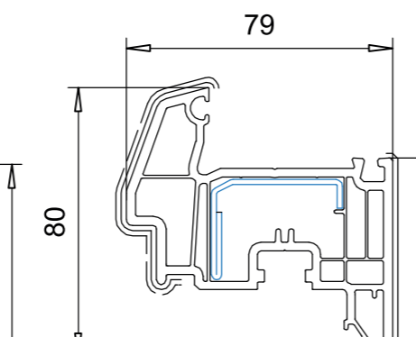
103.240 підсилювач 113.292 / 113.294 / 113.295
