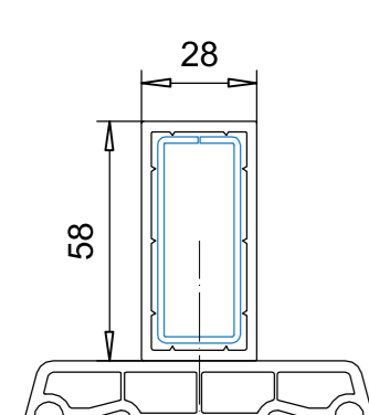
109.082 підсилювач 113.047.2
