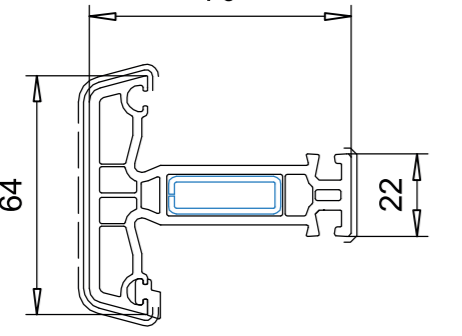
102.237 штульпова перекладина підсилювач 113.020
