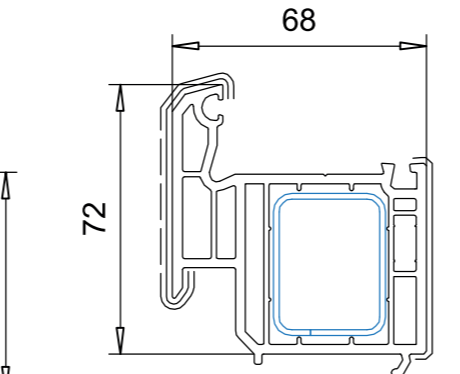
103.206 розширювальний профіль підсилювач 113.271
