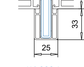
116.228.1 з ʼєднувач вертикальний підсилювач 113.149.2/ 113.120.3
