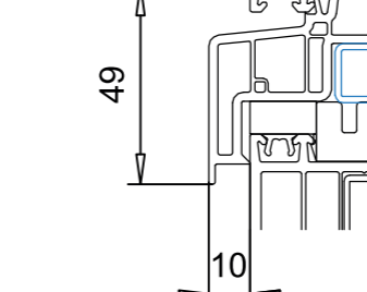
116.210 з ʼєднув. накладка підсилювач 113.347
