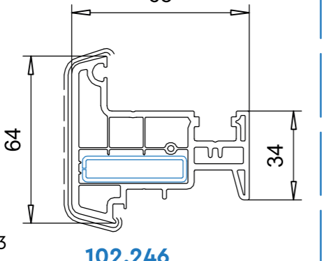
102.246 підсилювач 113.028
