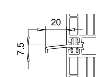
116.053 Міні з ʼєднувач
