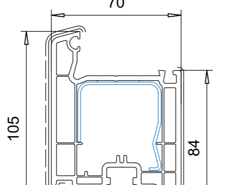
103.238 підсилювач 113.292 / 113.294 / 113.295
