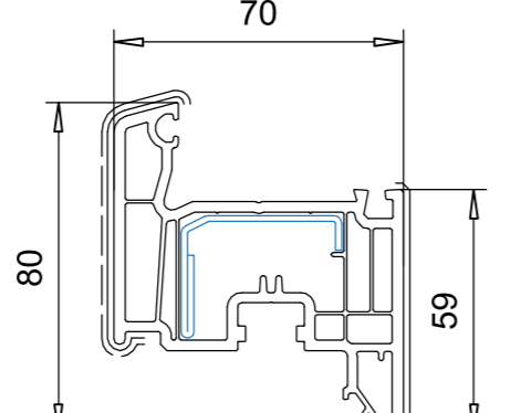
103.232 підсилювач 113.292 / 113.294 / 113.295
