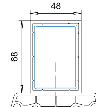
109.081 підсилювач 113.011.1, 113.001.2, 113.011.3
