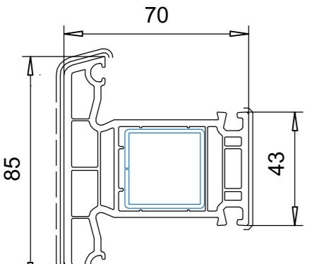
102.214 підсилювач 113.025
