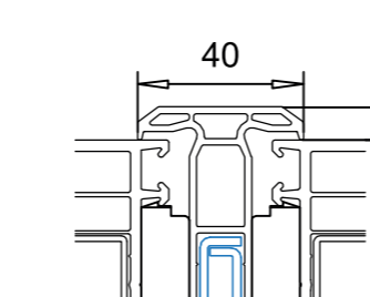
116.207 з ʼєднувач вертикальний підсилювач 113.149.2/ 113.120.3
