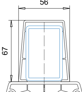
114.019 підсилювач 113.011.1/ 113.011.2/113.011.3
