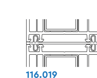
116.019 з ʼєднувальний профіль
