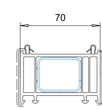
114.202 підсилювач 113.271/ 113.271.3
